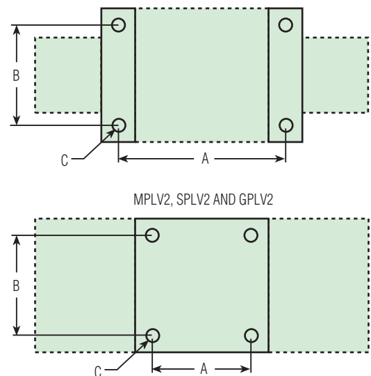
MOUNTING DIMENSIONS FOR AMPLIFIERS MPLV4-1, DLA5-1, DLA15-1, DLA30-1, MPLV2, DLA5 AND DLA15
